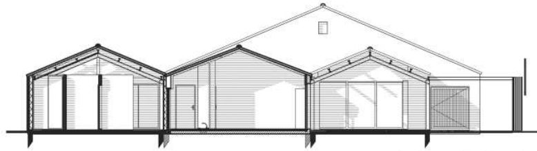
coupe de principe - échelle 1/100
